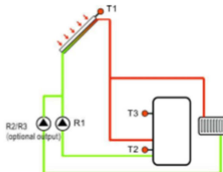
Funkce přenosu teplota pro čerpadlo
